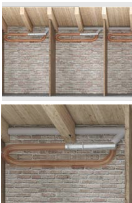
B Braccio flessibile con terminale di raccolta rigido
